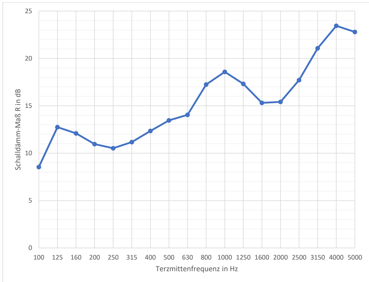
Abbildung 1: Rechnerisch simuliertes frequenzabhängiges Schalldämm-Maß R
